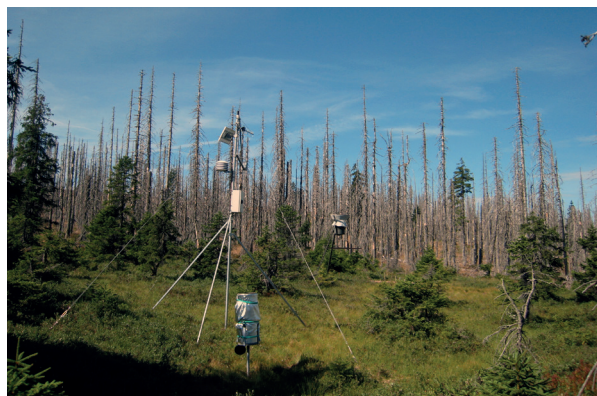
Obr. 4 Sněhoměrný polštář Plechý C7PLCH01, nadmořská výška 1 344 m n. m.
