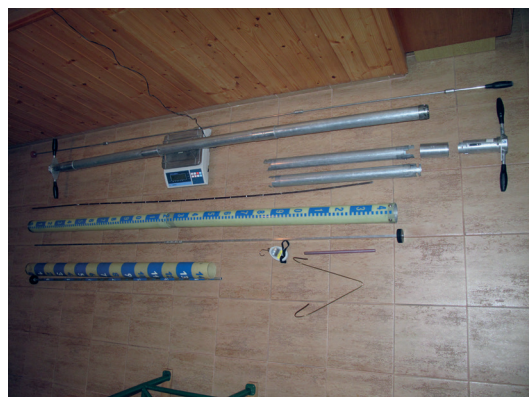
Obr. 4 Váhové sněhoměry používané na MS Lysá hora. Foto: 28. ledna 2019, Milan Čermák.
