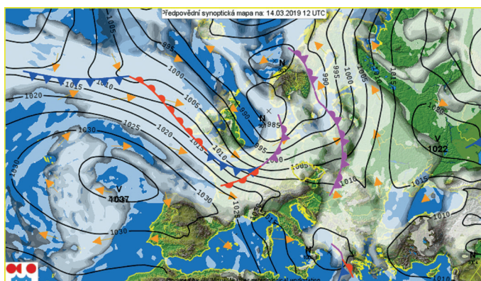
Obr. 1 Synoptická mapa. Zdroj: Předpovědní synoptická mapa Evropy, 2019.
