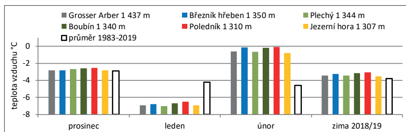
Obr. 2 Průměrná teplota vzduchu ( ^{\circ}\text{C} ) na hřebenu Šumavy v průběhu klimatologické zimy 2018/19 na vrcholových stanicích Grosser Arber, Březník hřeben, Plechý, Boubín, Poledník a Jezerní hora, v porovnání s dlouhodobým průměrem ze stanice Grosser Arber (1982–2018, Wetterzentrale 2019).
