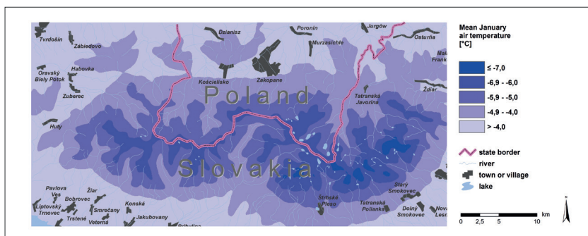
Obr. 3 Priemerná mesačná teplota vzduchu v januári za obdobie 1991–2010.
