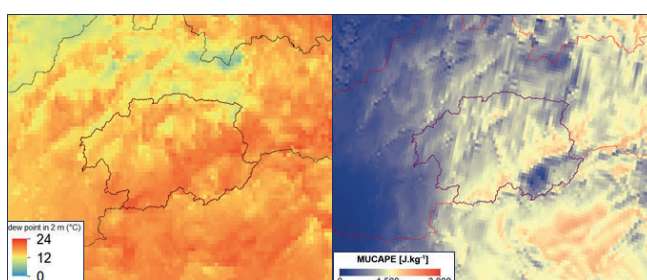
Obr. 1 Naľavo COSMO výpočet rozloženia teploty rosného bodu v 2m nad zemským povrchom (°C) a napravo most unstable CAPE (J.kg -1 ) nad Banskobystrickým krajom a priľahlým okolím 19. 07. 2011 v 12:00 SELČ.
